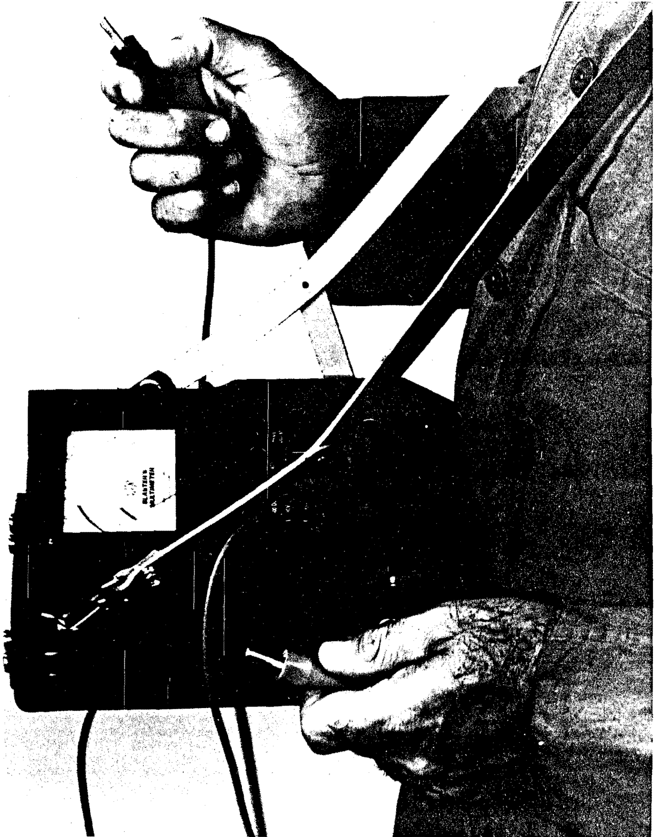
Figure 27.—Blasting multimeter. (Courtesy Du Pont Co.)
